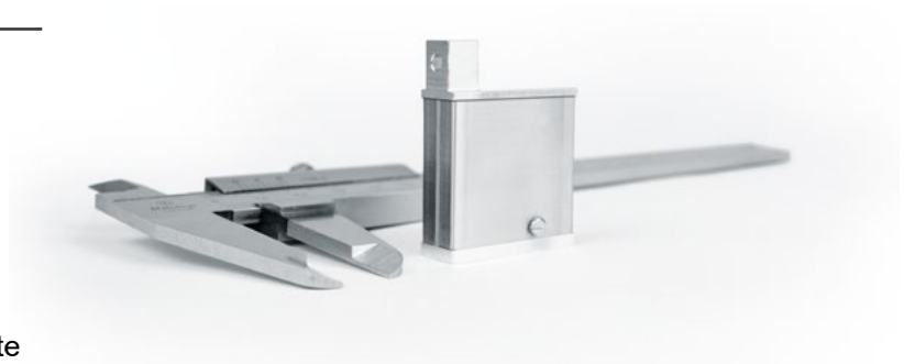
Fig. 1: MBB-01 Series | Capteur de force miniature (le calibre n'est pas inclus)
