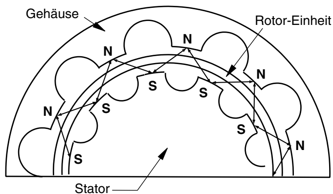
Bild 2. Struktur der Statorzähne
