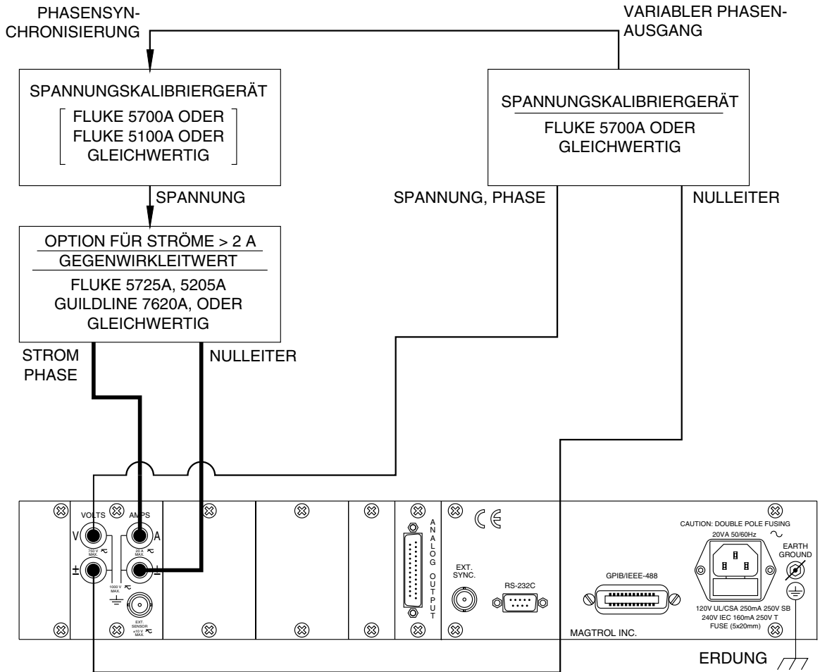
Bild 6–1 Prüfkfiguration zur Kalibrierung und Kontrolle
