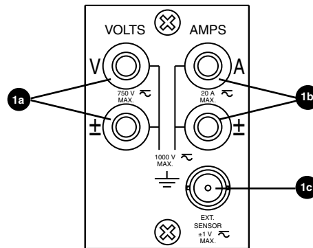
Bild 2-5 Eingangsmodul
