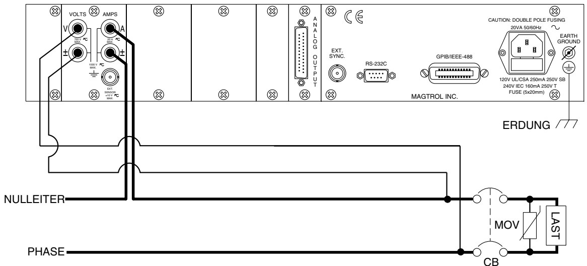
Bild 3-8 Einphasiger Anschluss (2 Leiter)
