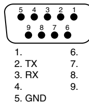
Bild 5–3 RS-232-Schnittstelle
