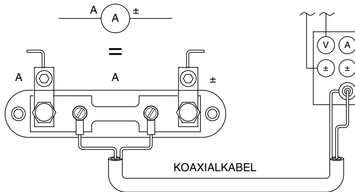
Bild 3-9 Anschlusschema mit Aufnehmer
