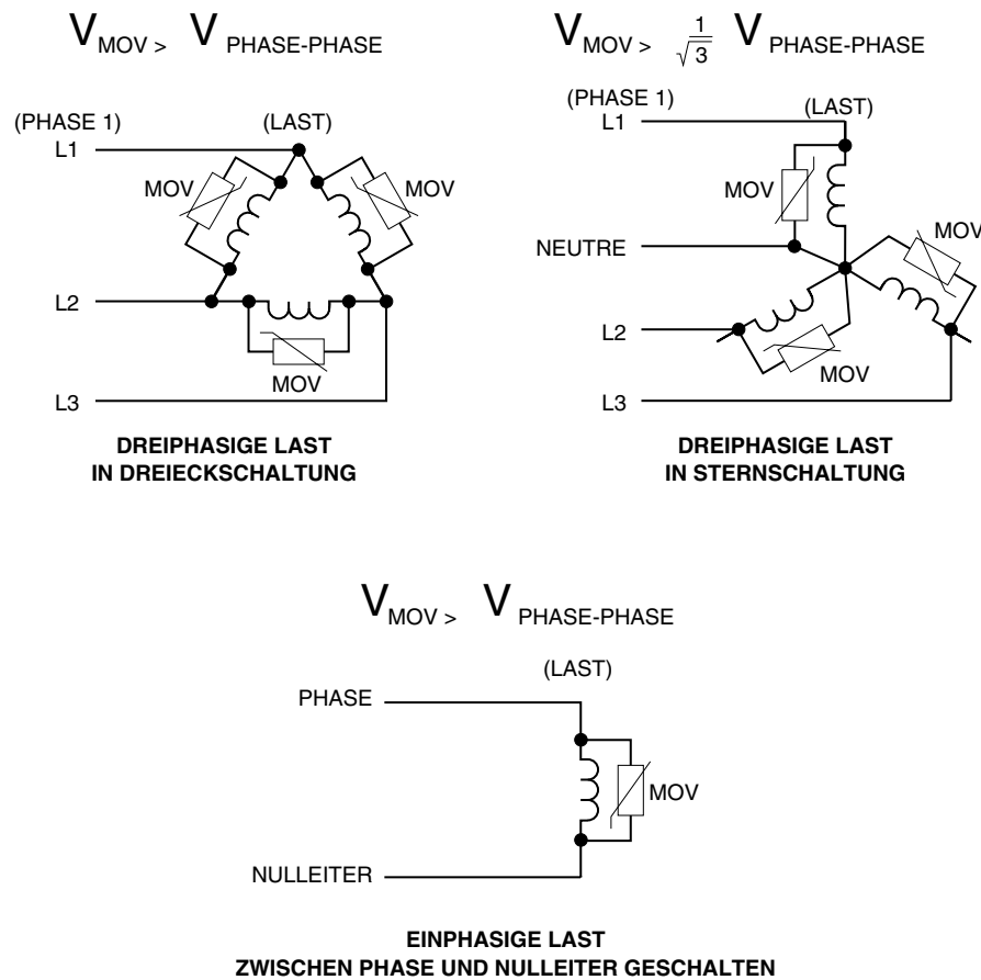
Bild 3–6 Unterdrückung transienter Spannungen
