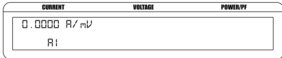
Bild 3–11 Konfigurationsmenü des Skalierungsfaktors des externen Aufnehmers
