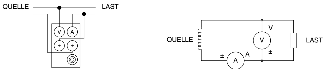
Bild 3-7 Schema eines einphasigen Messsystems (2 Leiter)
