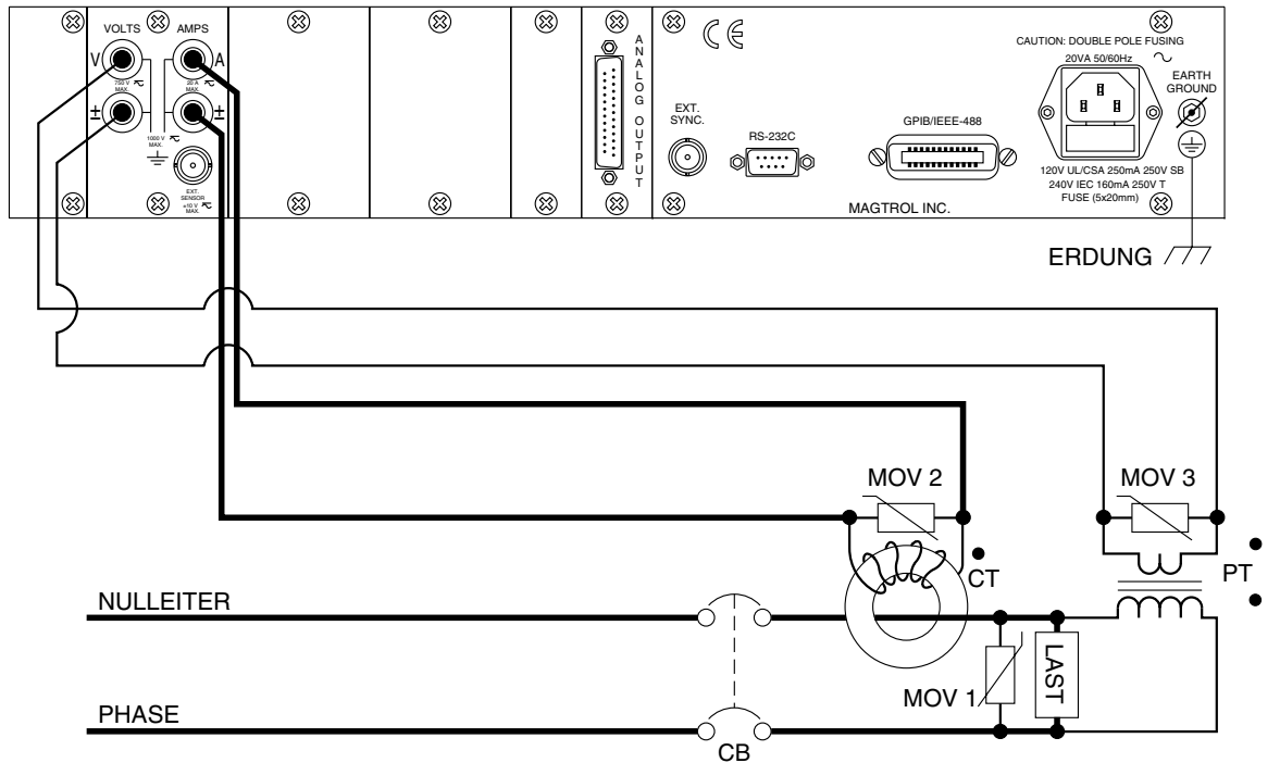
Bild 3–12 Anschluss des Strom-/Spannungswandlers
