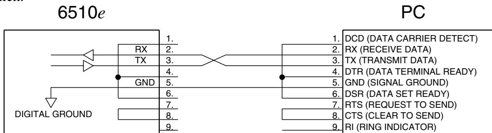
Bild 5–4 Null-Modem-Kabelanschluss
