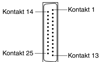
Bild 7-1 Analogausgänge
