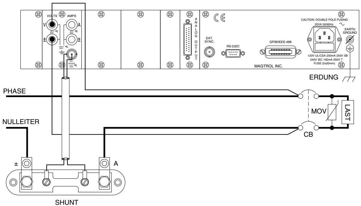
Bild 3-10 Anschluss des externen Aufnehmers
